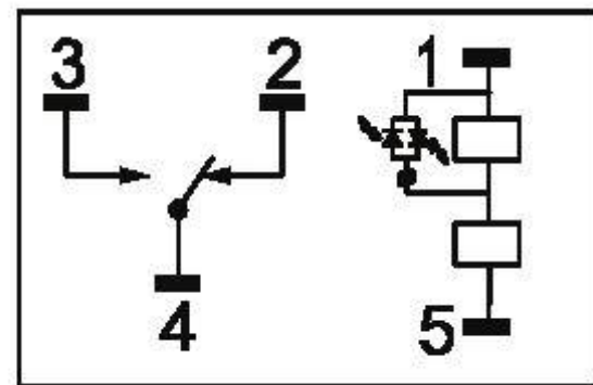
LED(DC)
