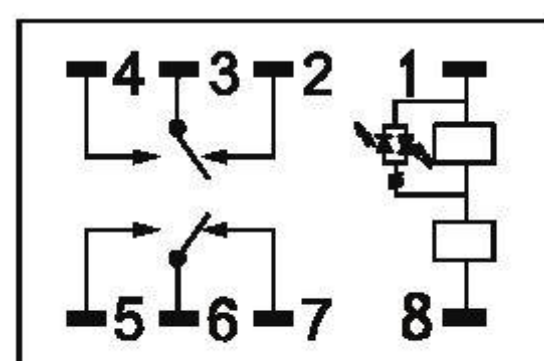
LED(DC)
