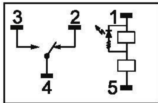
LED(AC)
