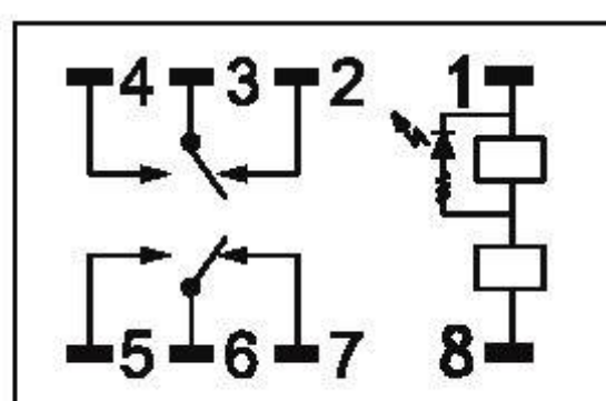
LED(AC)
